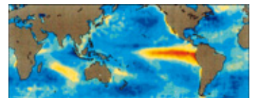
Anomale Meeresoberflächentemperatur, beobachtet während des letzten starken El Niños.
